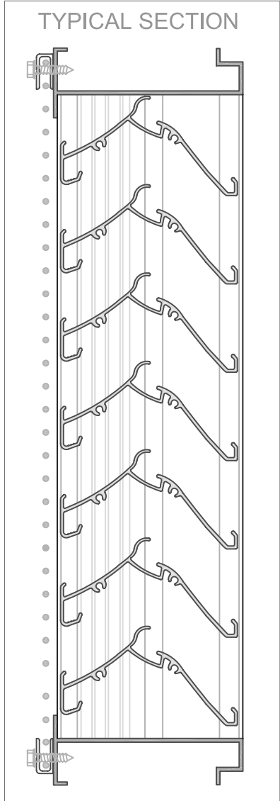
AA - LOUVER SECTION
